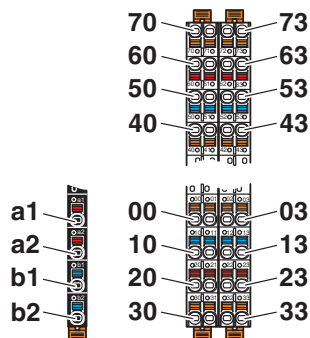
Bild 2 Klemmpunktbelegung
