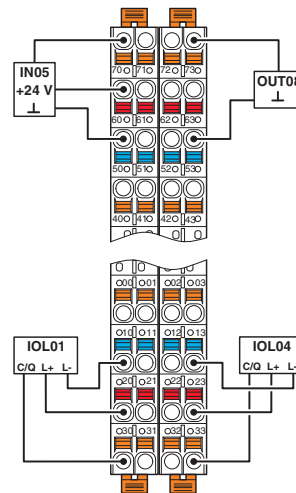
Bild 3 Anschlussbeispiel
