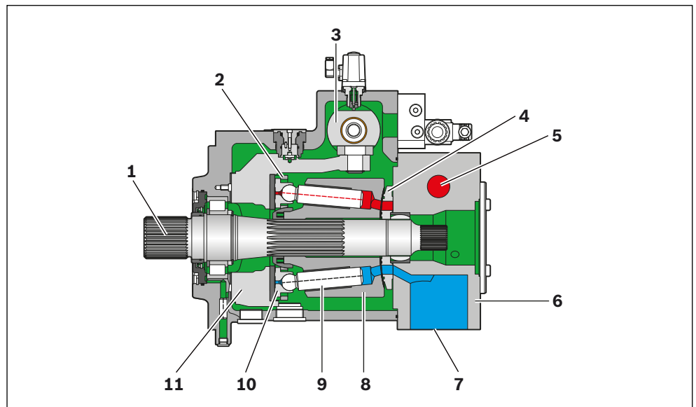
Abb. 2: Aufbau der A4VBO
