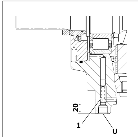
Abb. 9: Drosselschraube Nenngröße 450
