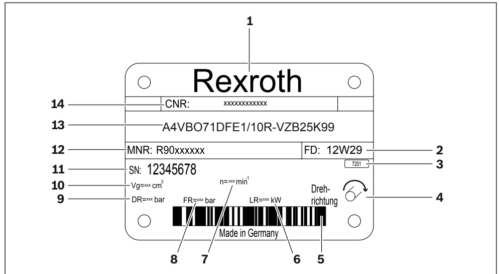
Abb. 3: Typschild A4VBO
