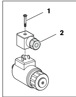
Abb. 17: Anziehdrehmoment Hirschmann-Stecker
