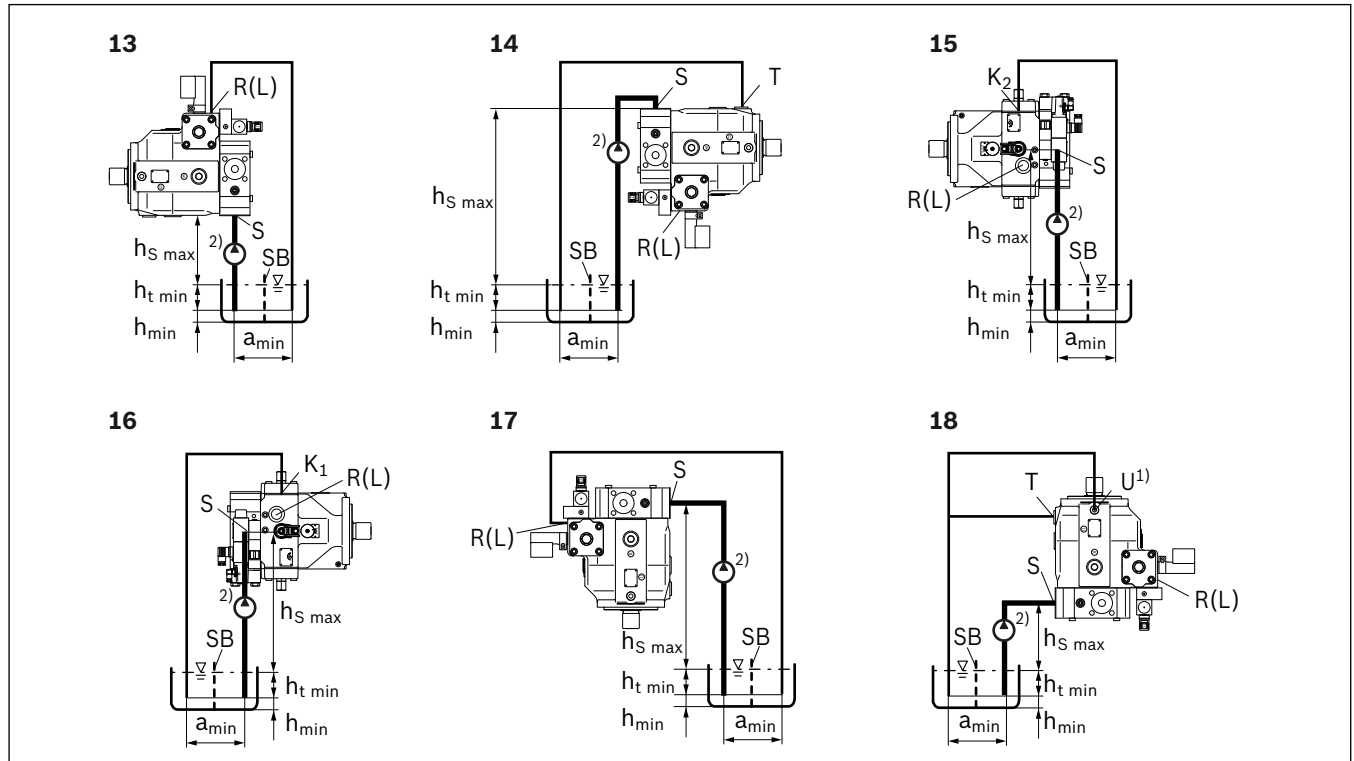
Abb. 12: Untertankeinbau A4VBO mit Einbaulage 13–18
