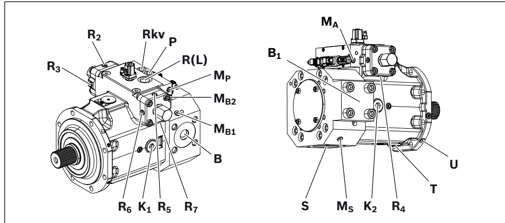
Abb. 15: Anschlussübersicht A4VBO, HS4-Regelsystem mit Proportionalventil, Nenngröße 450
