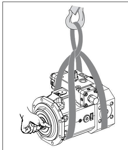
Abb. 6: Transport mit Hebeband
