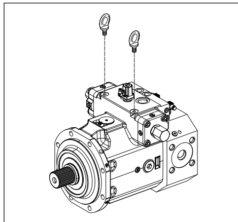
Abb. 5: Befestigung der Ringschrauben im Gehäuse
