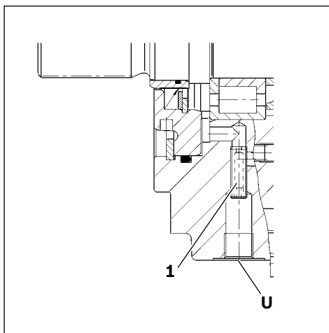
Abb. 8: Drosselschraube Nenngroße 125
