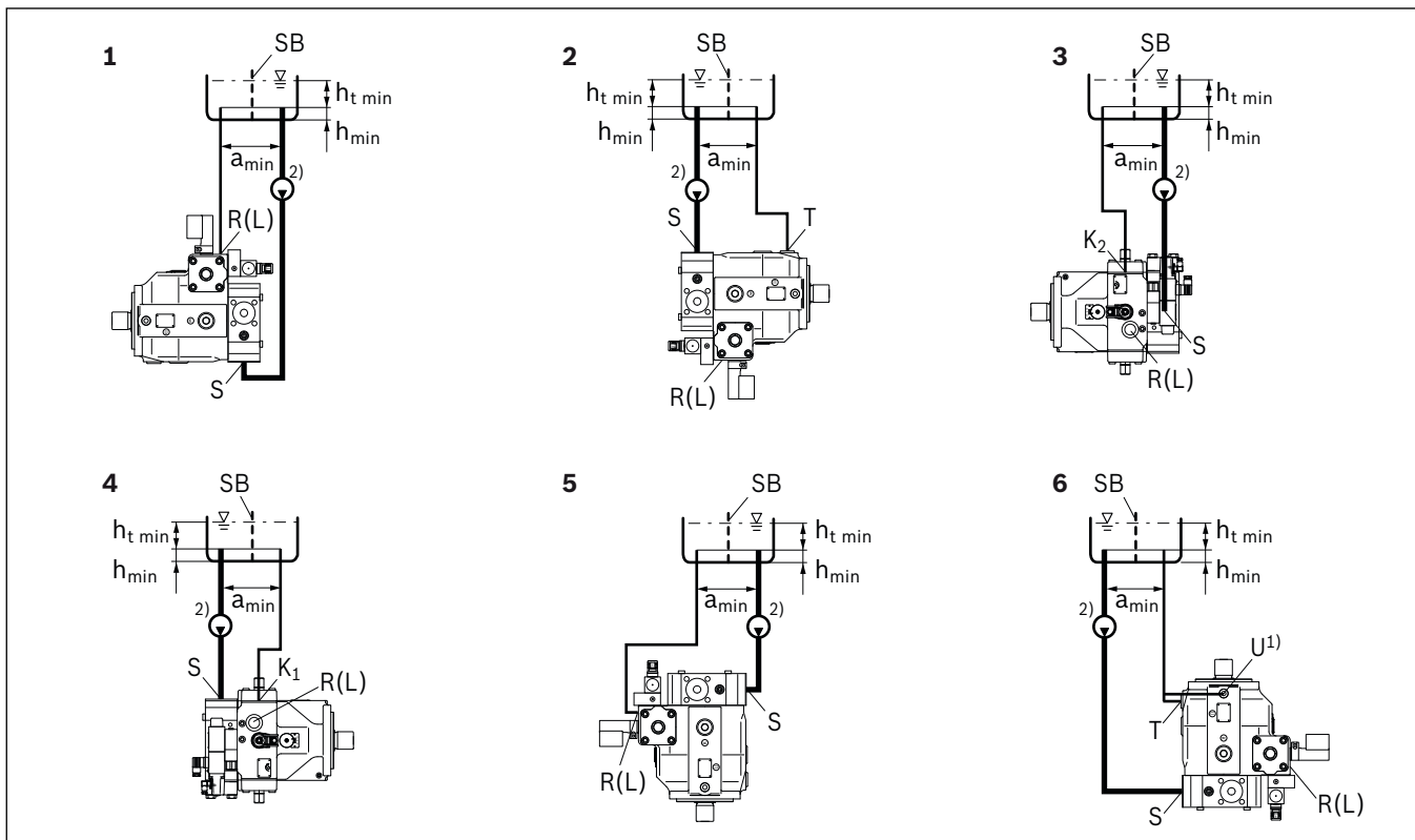
Abb. 10: Untertankeinbau A4VBO mit Einbaulage 1–6
