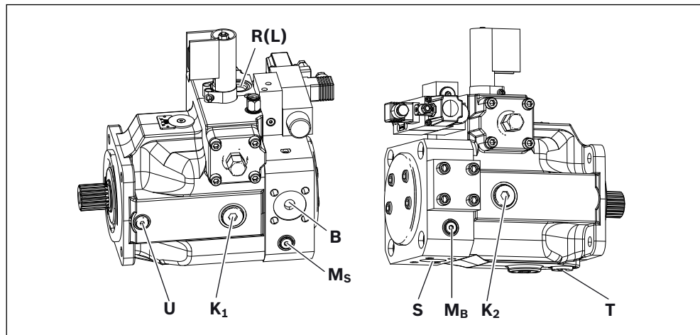
Abb. 16: Anschlussübersicht A4VBO, DFE1-Elektro-hydraulisches Regelsystem, Nenngröße 71
