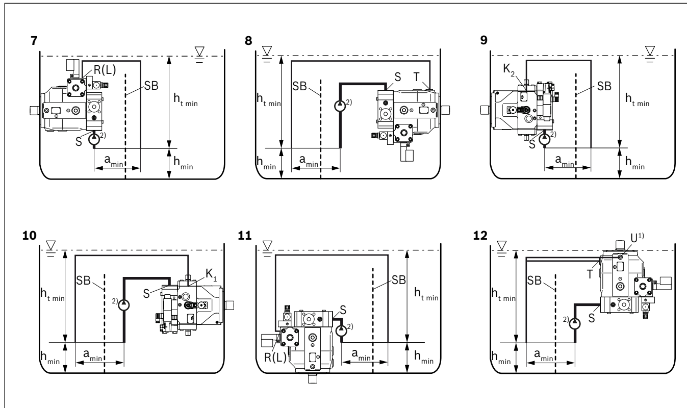
Abb. 11: Tankeinbau A4VBO mit Einbaulage 7-12
