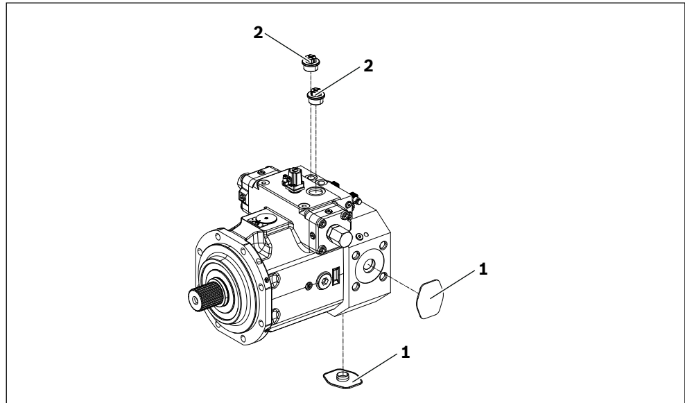
Abb. 1: Axialkolbeneinheit
