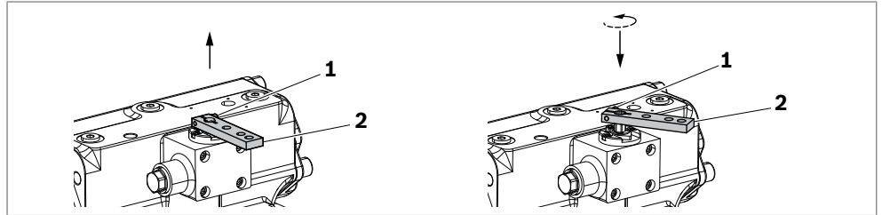
Abb. 12: Hebelposition von HW-Verstellung ändern
