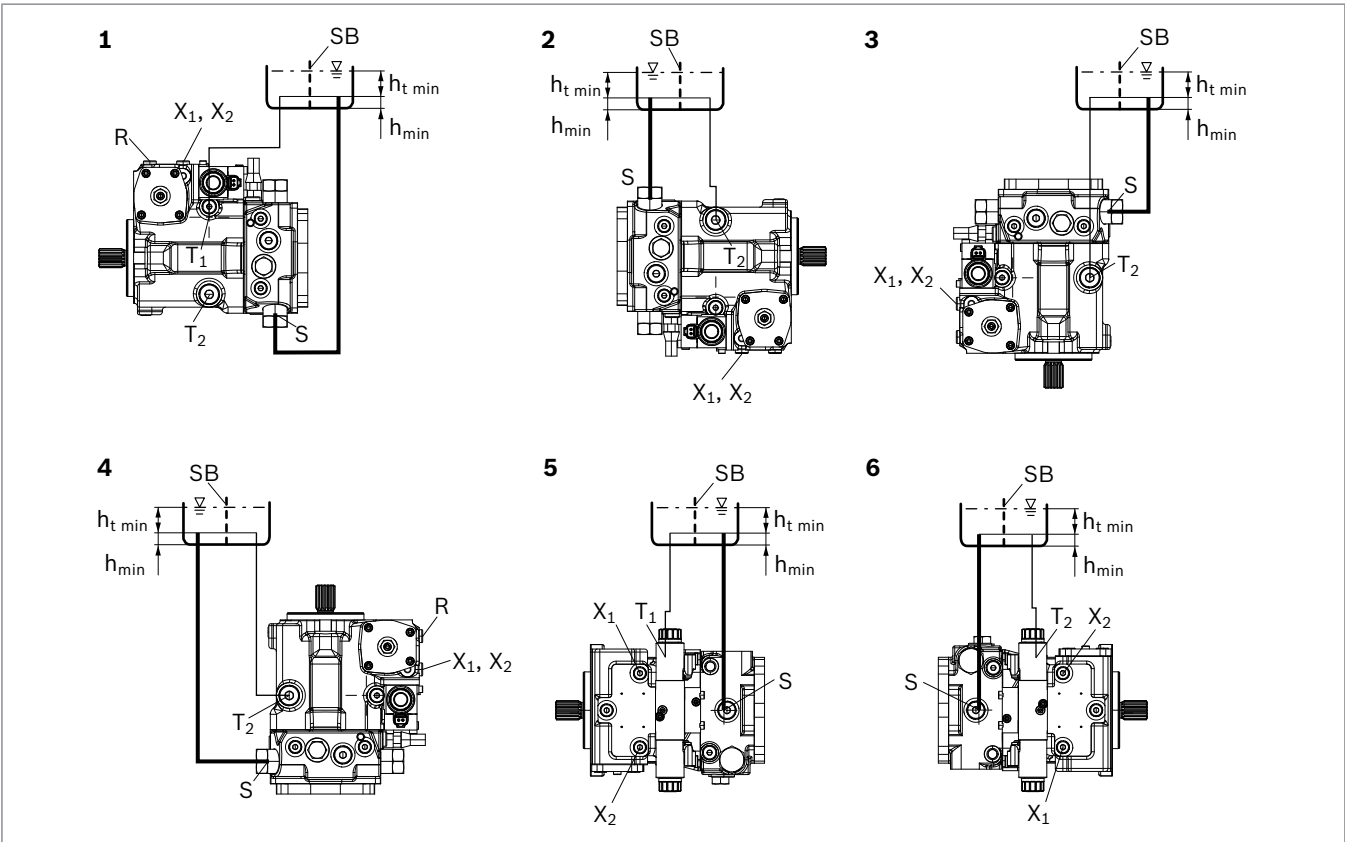
Abb. 8: Untertankeinbau mit Einbaulage 1-6
