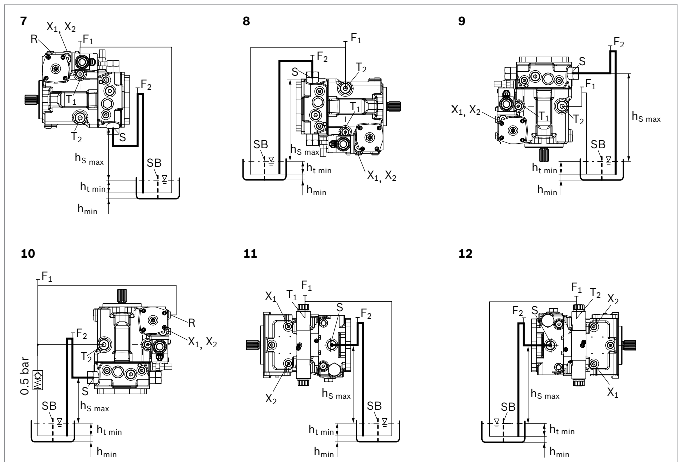
Abb. 9: Übertankeinbau mit Einbaulage 7-12
