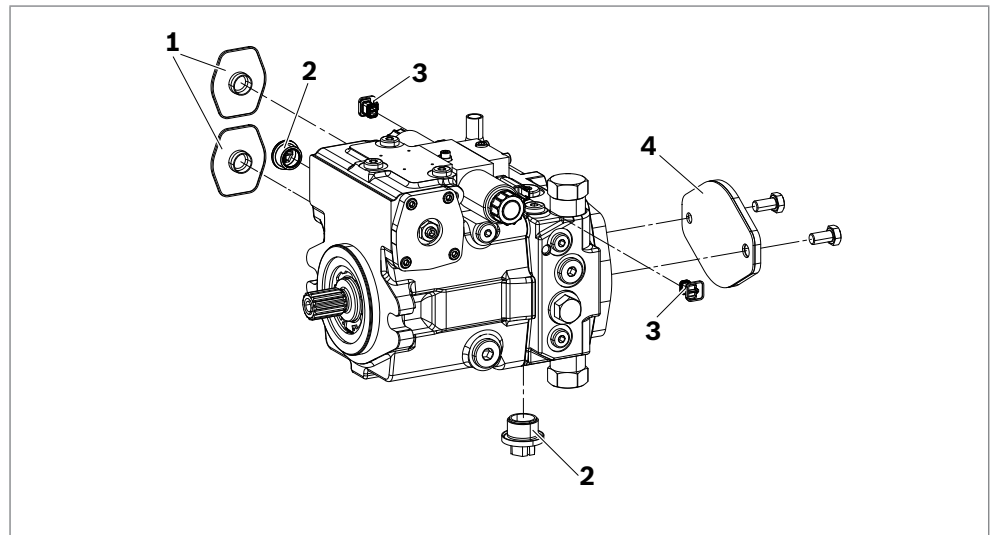
Abb. 1: Axialkolbeneinheit
