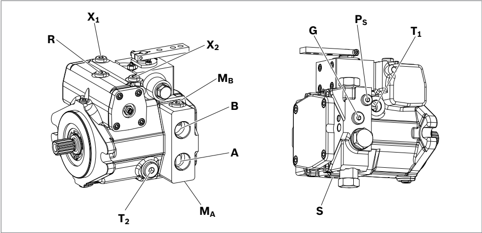
Abb. 14: Anschlussübersicht Nenngröße 18
