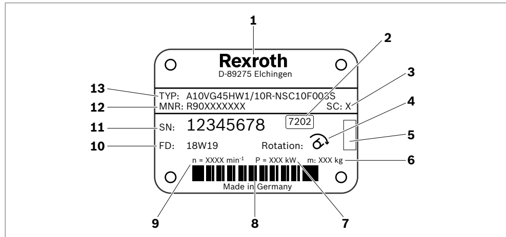
Abb. 4: Typschild A10VG
