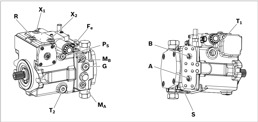
Abb. 15: Anschlussübersicht Nenngröße 28 und 45
