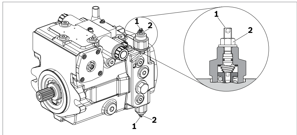
Abb. 3: Bypass-Funktion aktivieren
