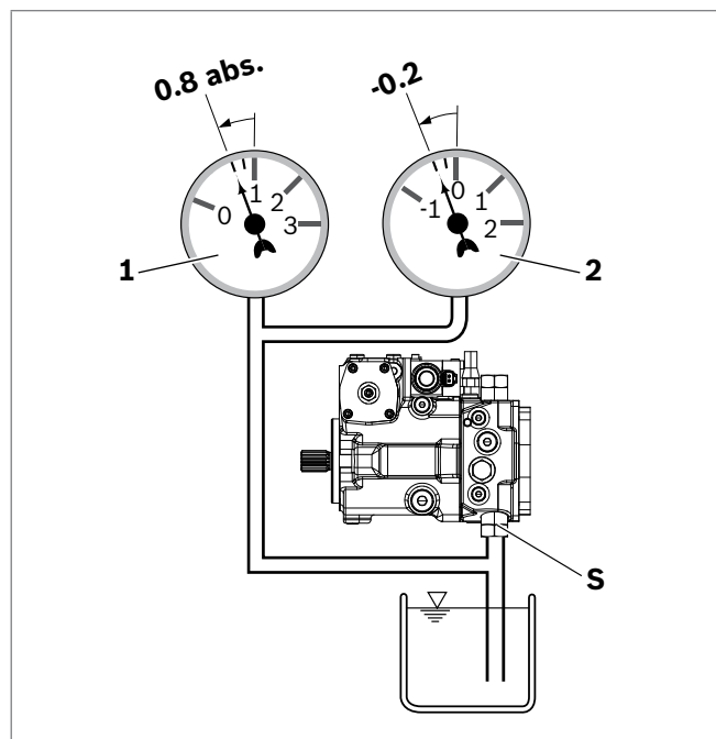
Abb. 7: Saugdruck
