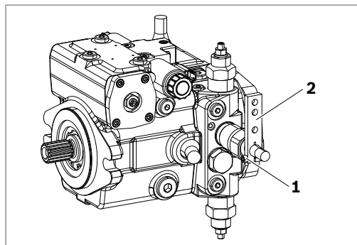
Abb. 13: Hebelposition von DA-Regelventil ändern
