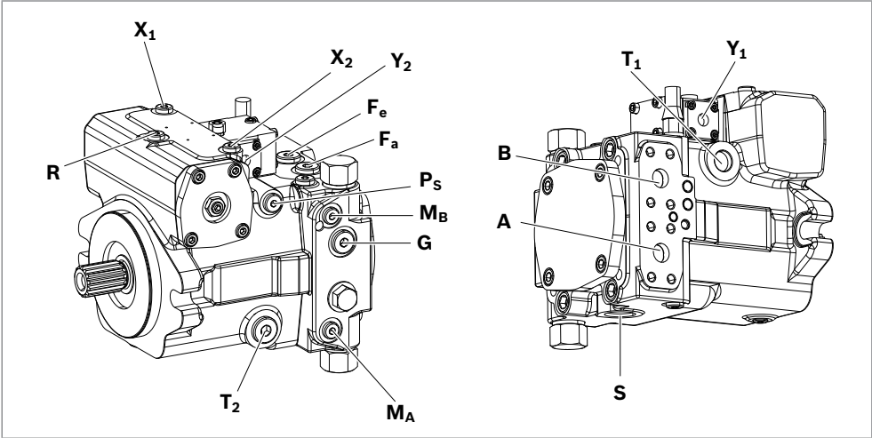
Abb. 16: Anschlussübersicht Nenngröße 63
