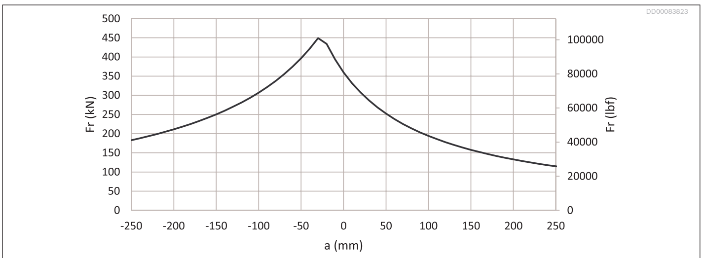
Fig. 40: Permissible external static load Häggglunds Atom 40
